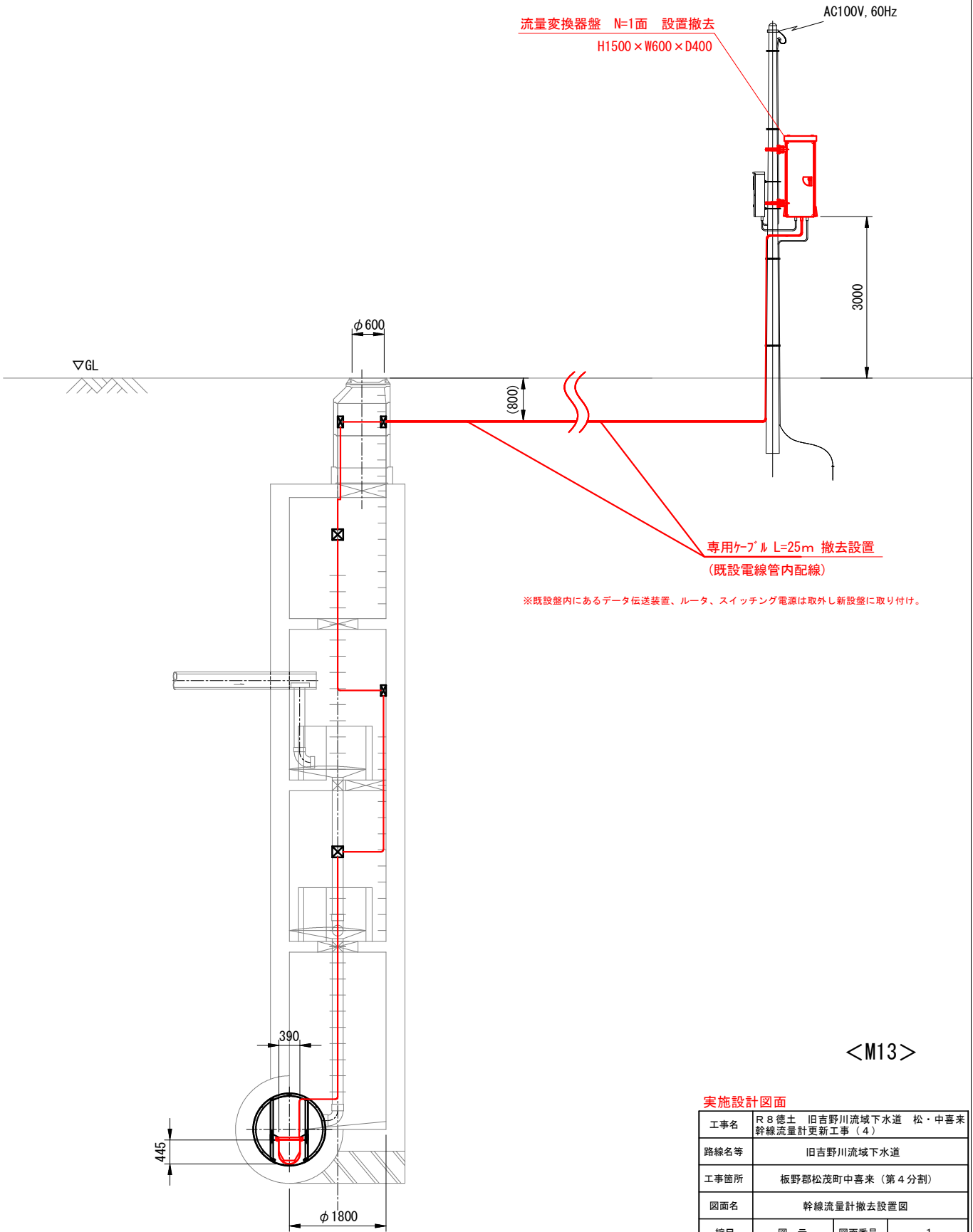
B-B断面図
