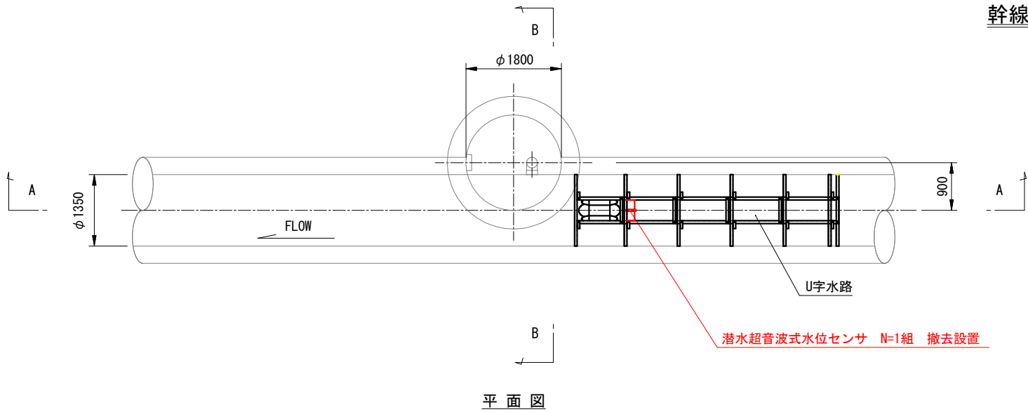
平面図
