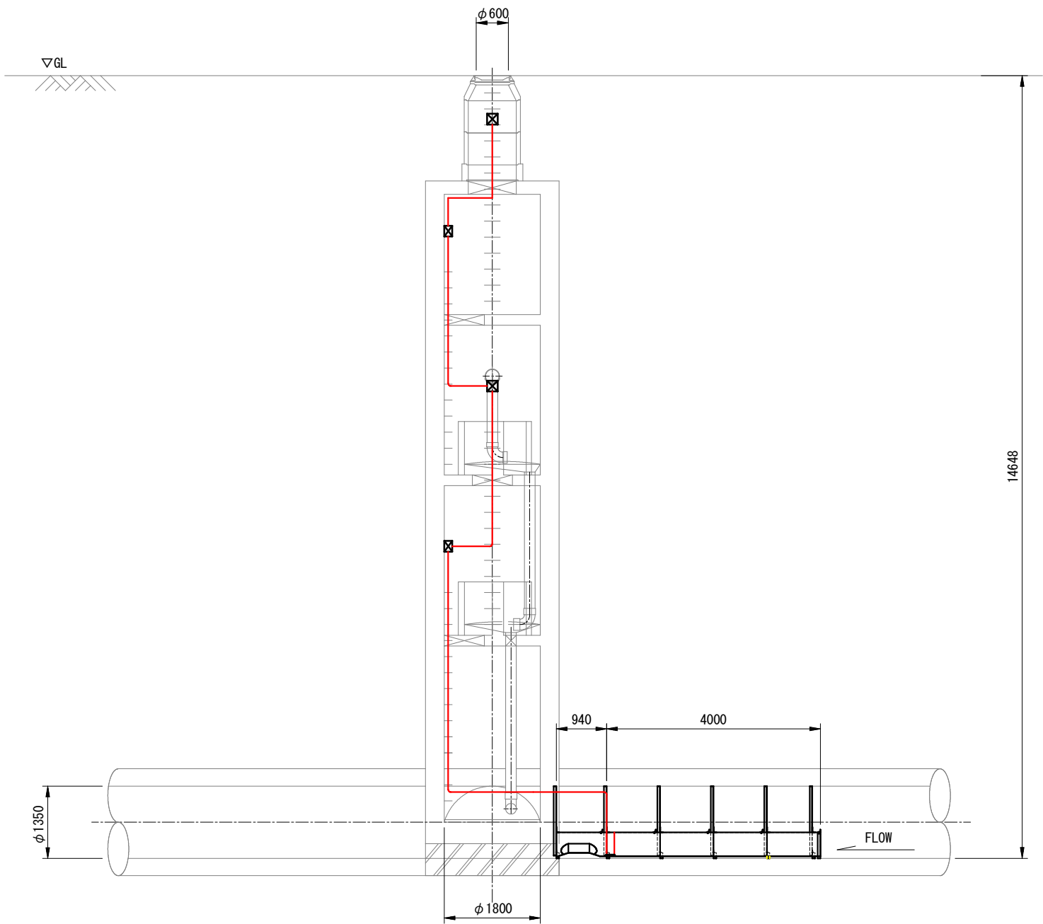
A-A断面図
